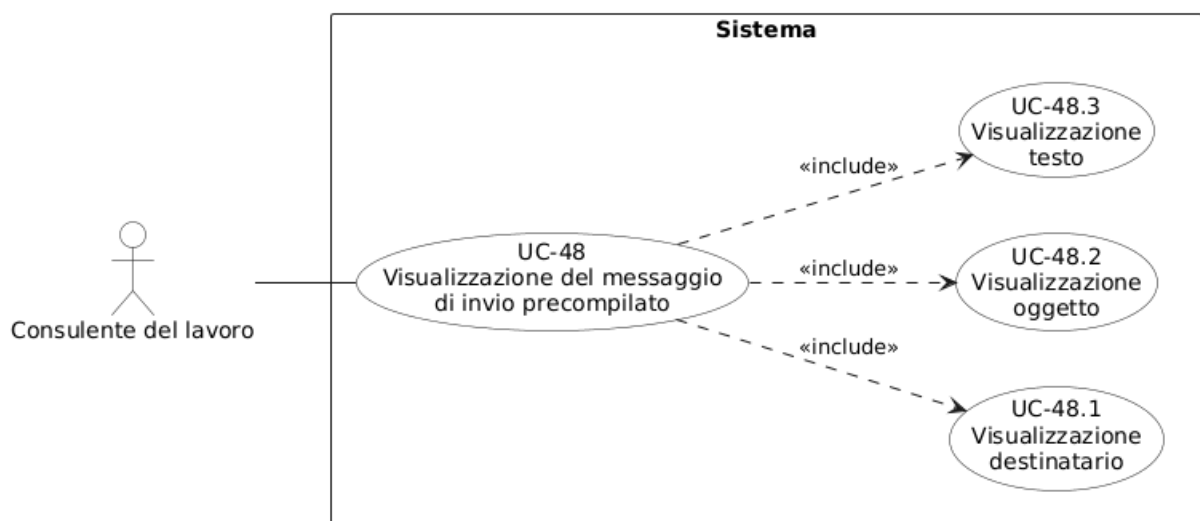
Figura 69: Diagramma del caso d'uso UC-48: Visualizzazione del messaggio di invio precompilato
